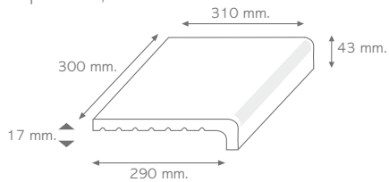
Peldaño Recto 31 x 30 cm.
