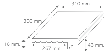
Peldaño Paloma 31 x 30 cm.
