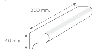
Esquina 4 x 30 cm.
