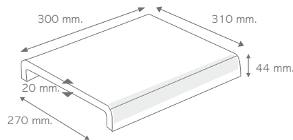
Pasamanos Fiorentino 31 x 30 cm.
