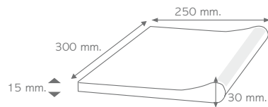
Borde Piscina 25 x 30 cm.
